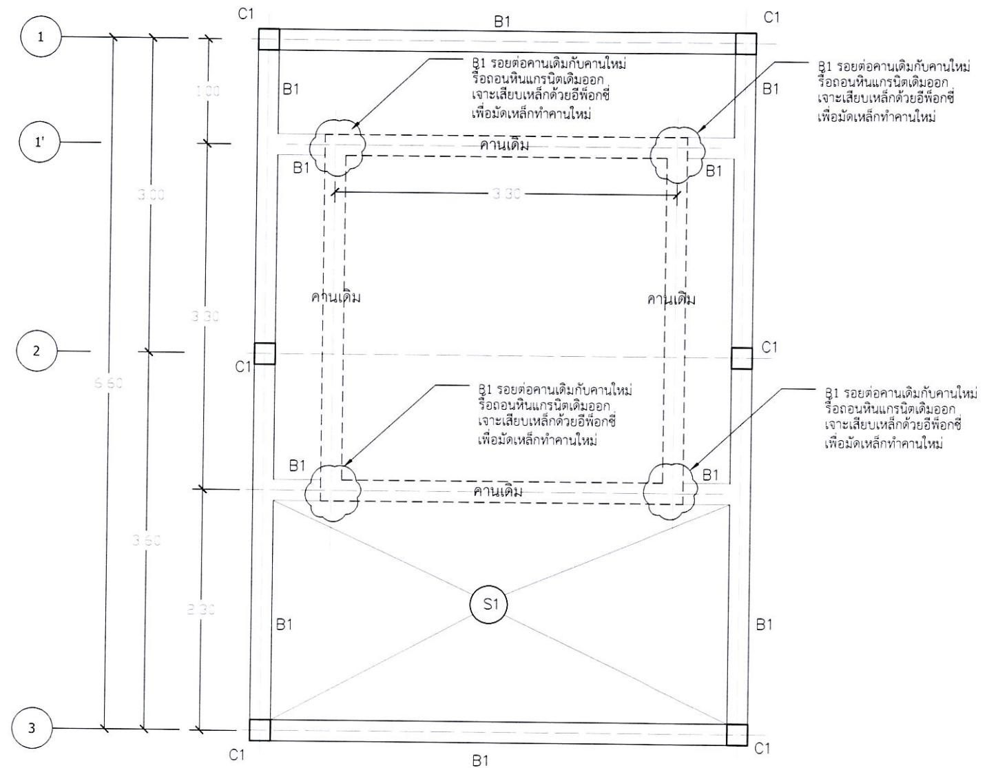
แปลนคานคอดิน มาตราส่วน 1 : 50
