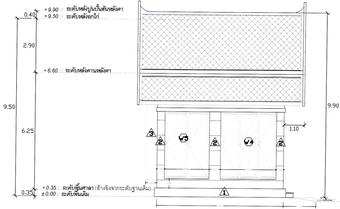
รูปด้านข้าง Scale: 1:100
