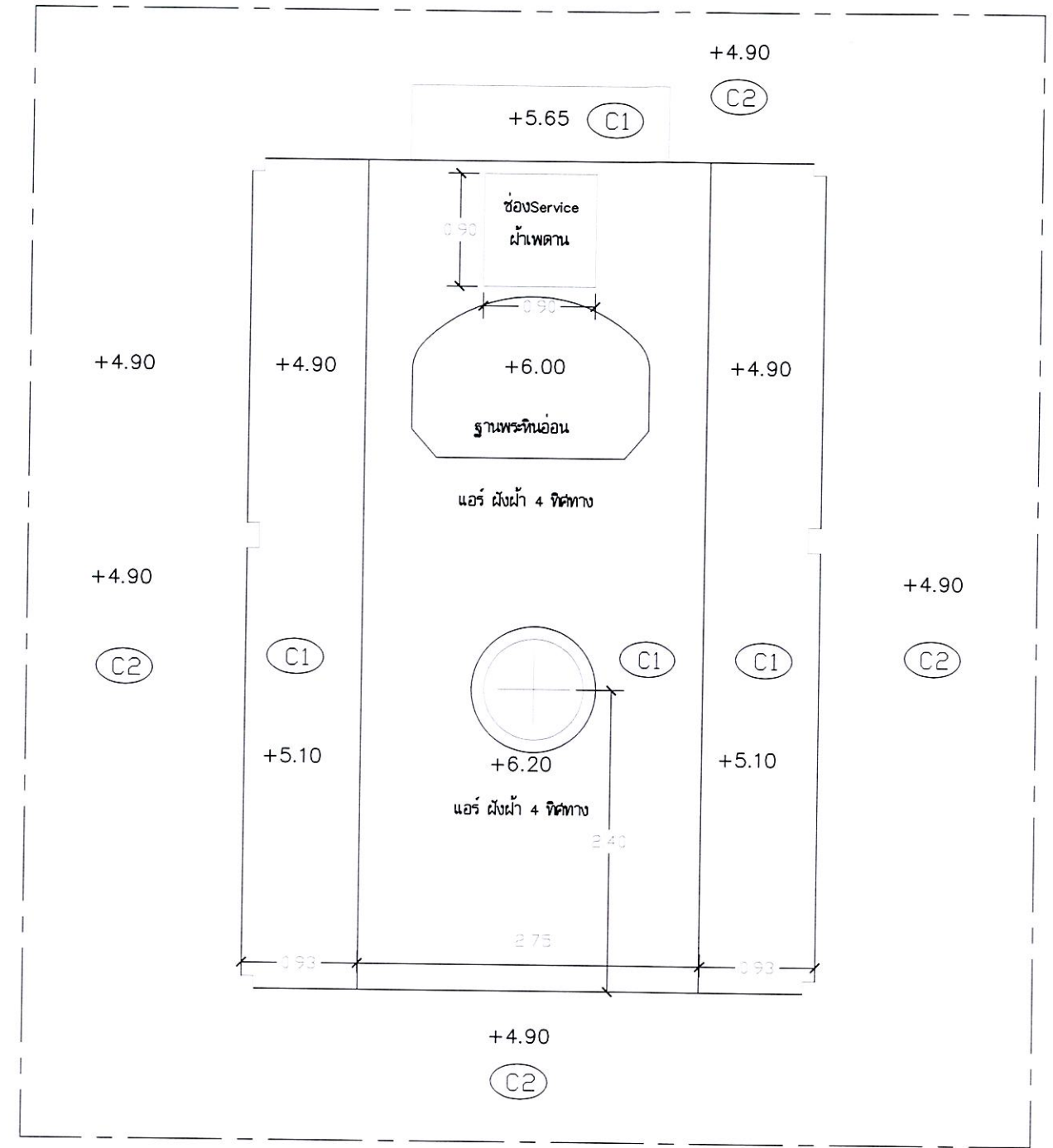
แปลนผ้าเพดาน 1:50
