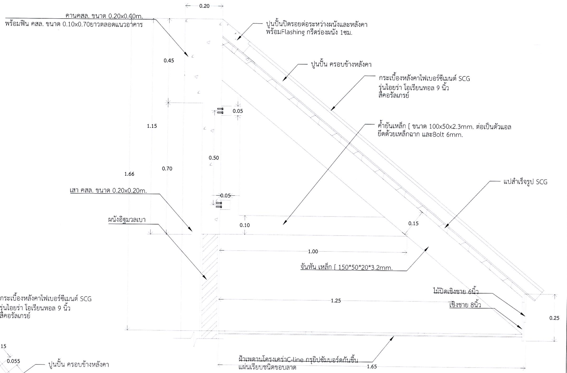
แบบขยาย 1 เหล็กค้ำหลังคาชั้นล่าง 1:10
