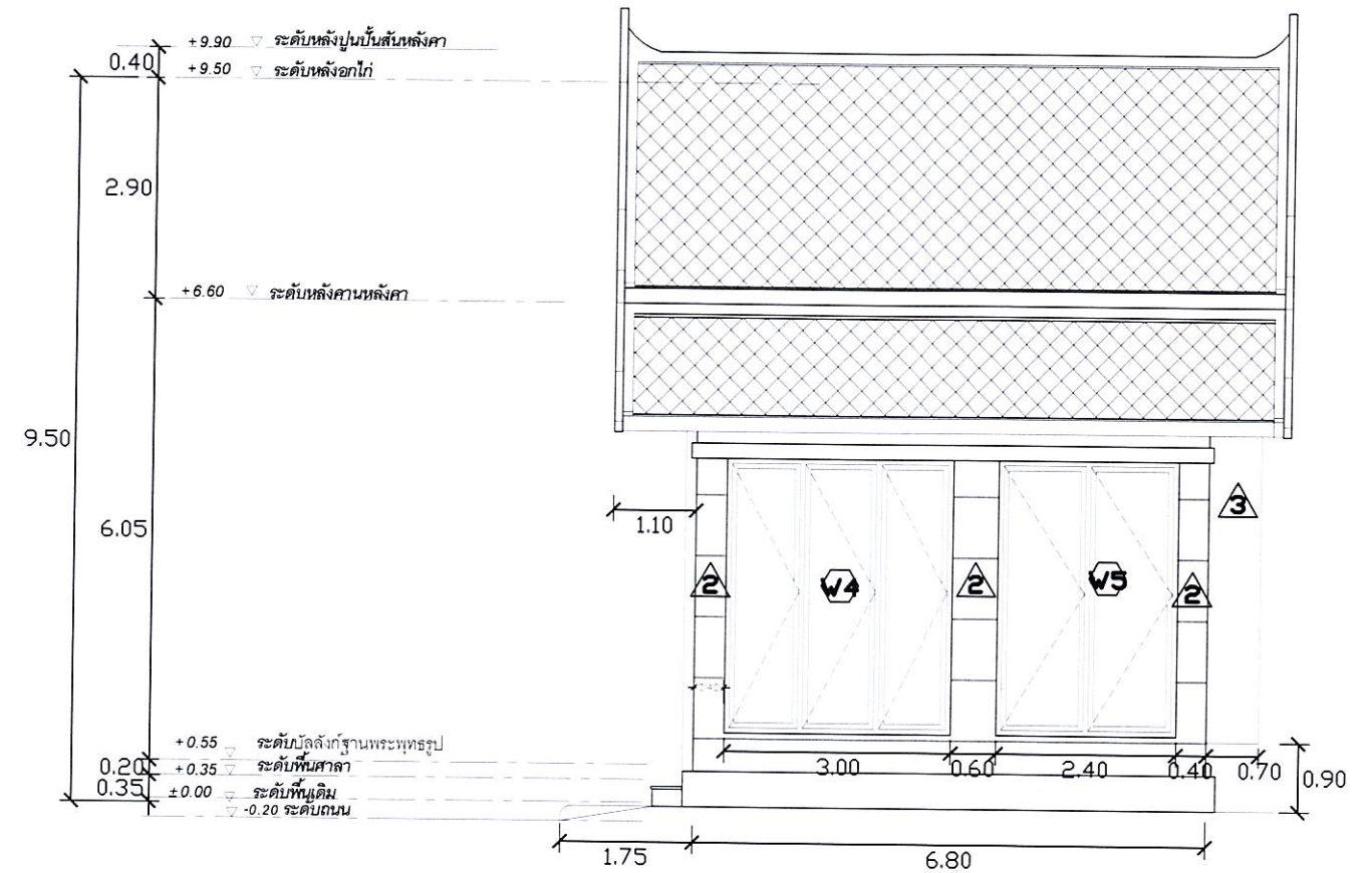
รูปด้านข้าง Scale: 1:100
