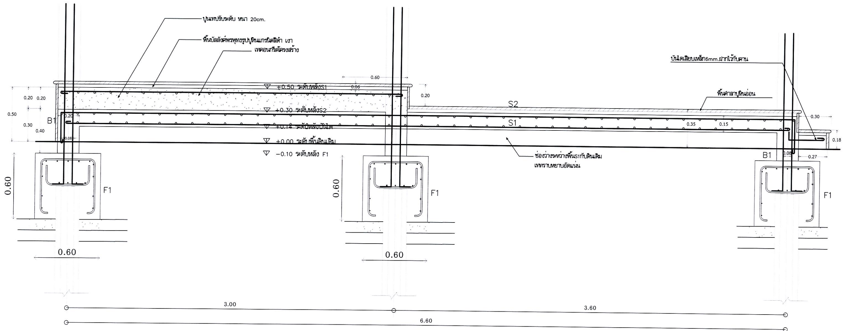
แปลนฐานราก F1 1:20
