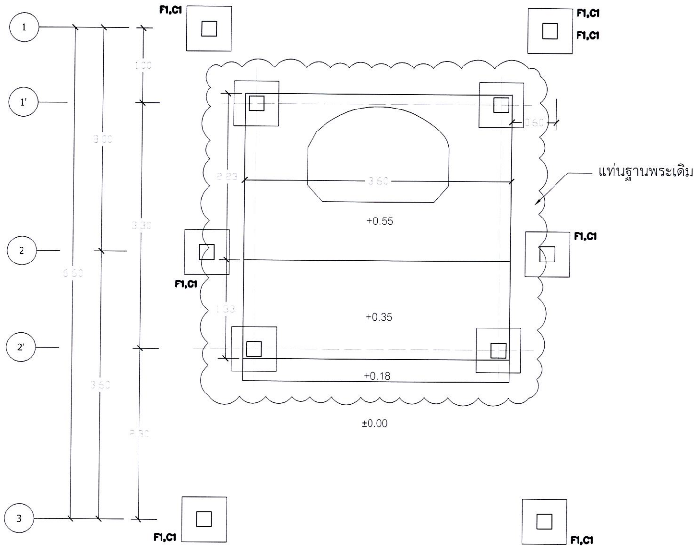
แปลนฐานราก ต่อม่อ มาตราส่วน 1 : 50
