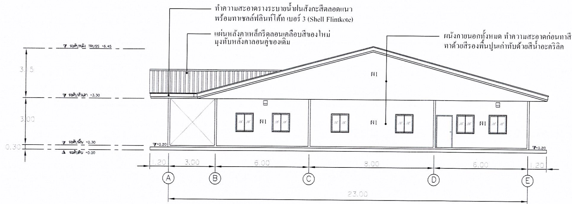
รูปด้าน D อาคารที่ทำการสหภาพแรงงานรัฐวิสาหกิจฯ
