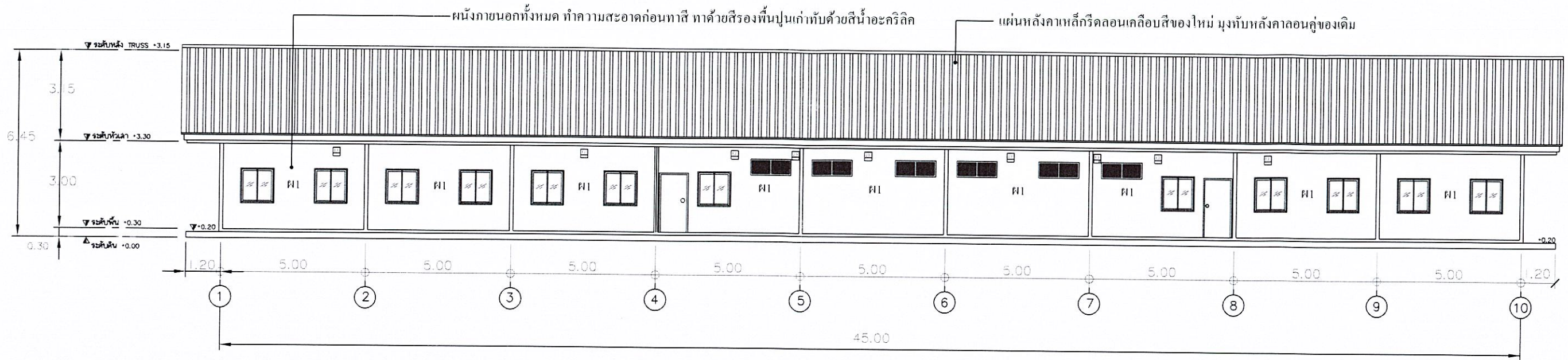
รูปด้าน C อาคารที่ทำการสหภาพแรงงานรัฐวิสาหกิจฯ
