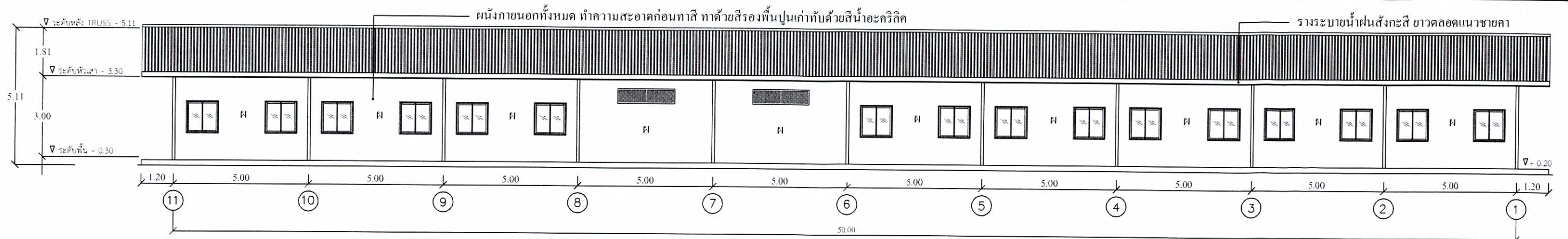
รูปด้าน C อาคารสำนักงานโครงการ 1 : 150
