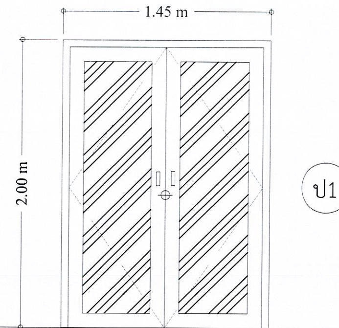
รูปประตูบานเปิดคู่วงกบ-กรอบบานอะลูมิเนียมกระจกใส มาตราส่วน 1 : 25
