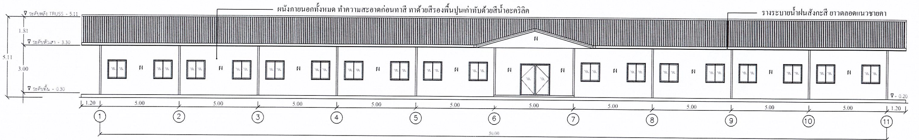
รูปด้าน A อาคารสำนักงานโครงการ 1 : 150
