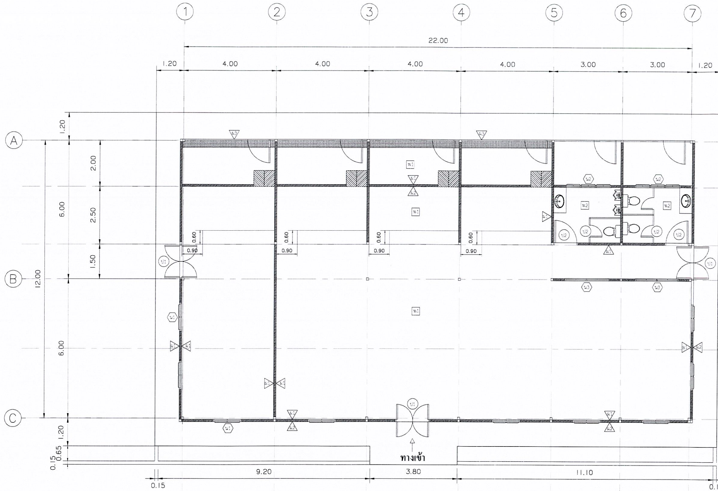
แปลนพื้นอาคารโรงอาหารชั่วคราว มาตรฐาน 1 : 100
