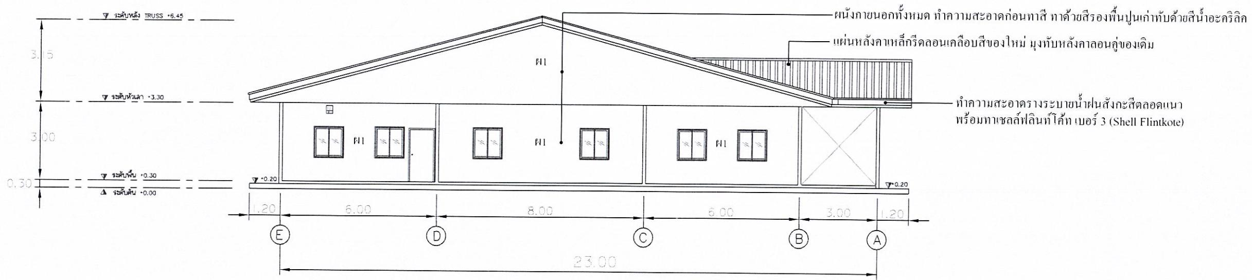
รูปด้าน B อาคารที่ทำการสหภาพแรงงานรัฐวิสาหกิจฯ 1 : 150
