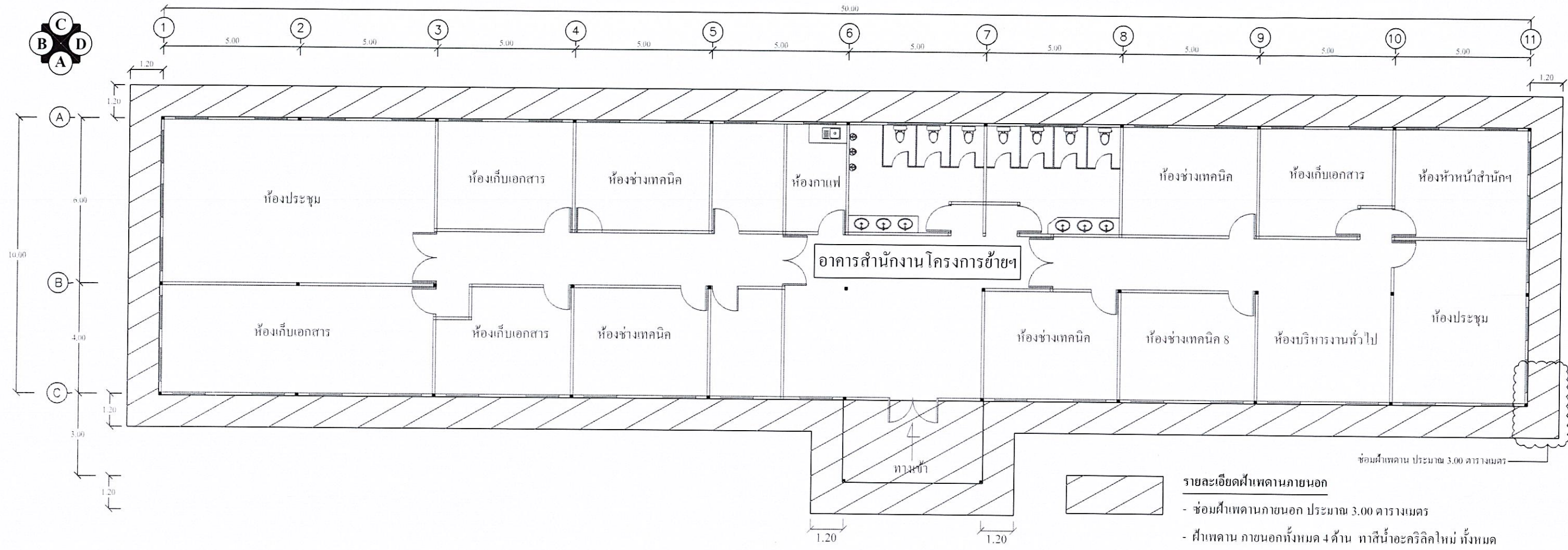
แปลน พื้นเพดานภายนอก อาคารสำนักงานโครงการฯ 1 : 150
