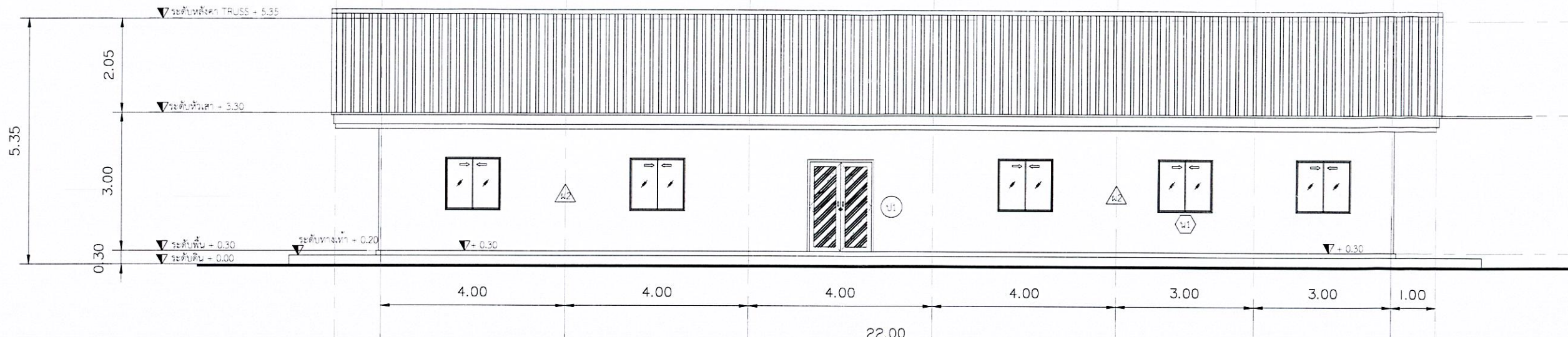
รูปด้านอาคารโรงอาหารชั่วคราว 1 4-001 1 : 100
