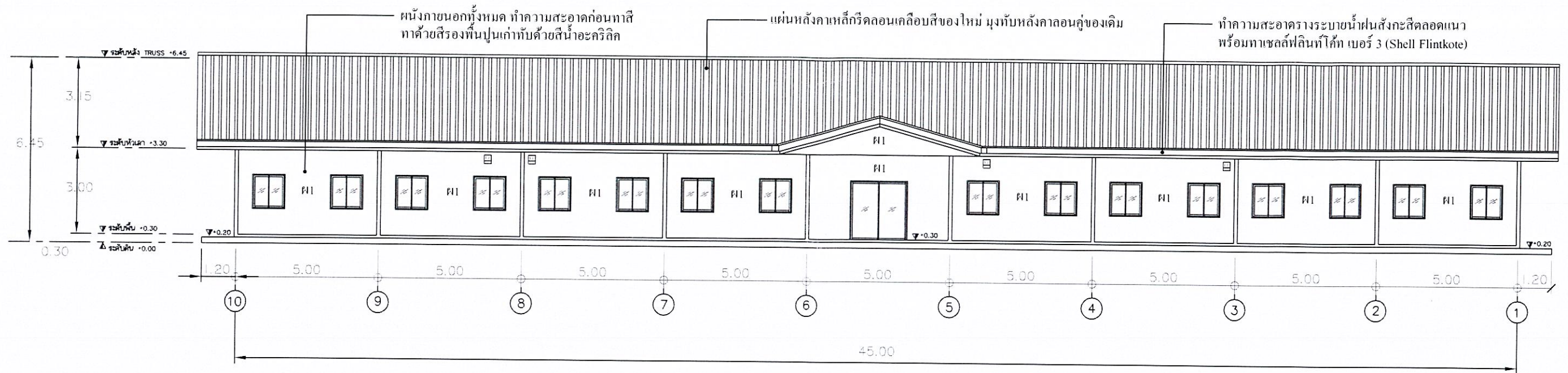
รูปด้าน A อาคารที่ทำการสหภาพแรงงานรัฐวิสาหกิจฯ 1 : 150
