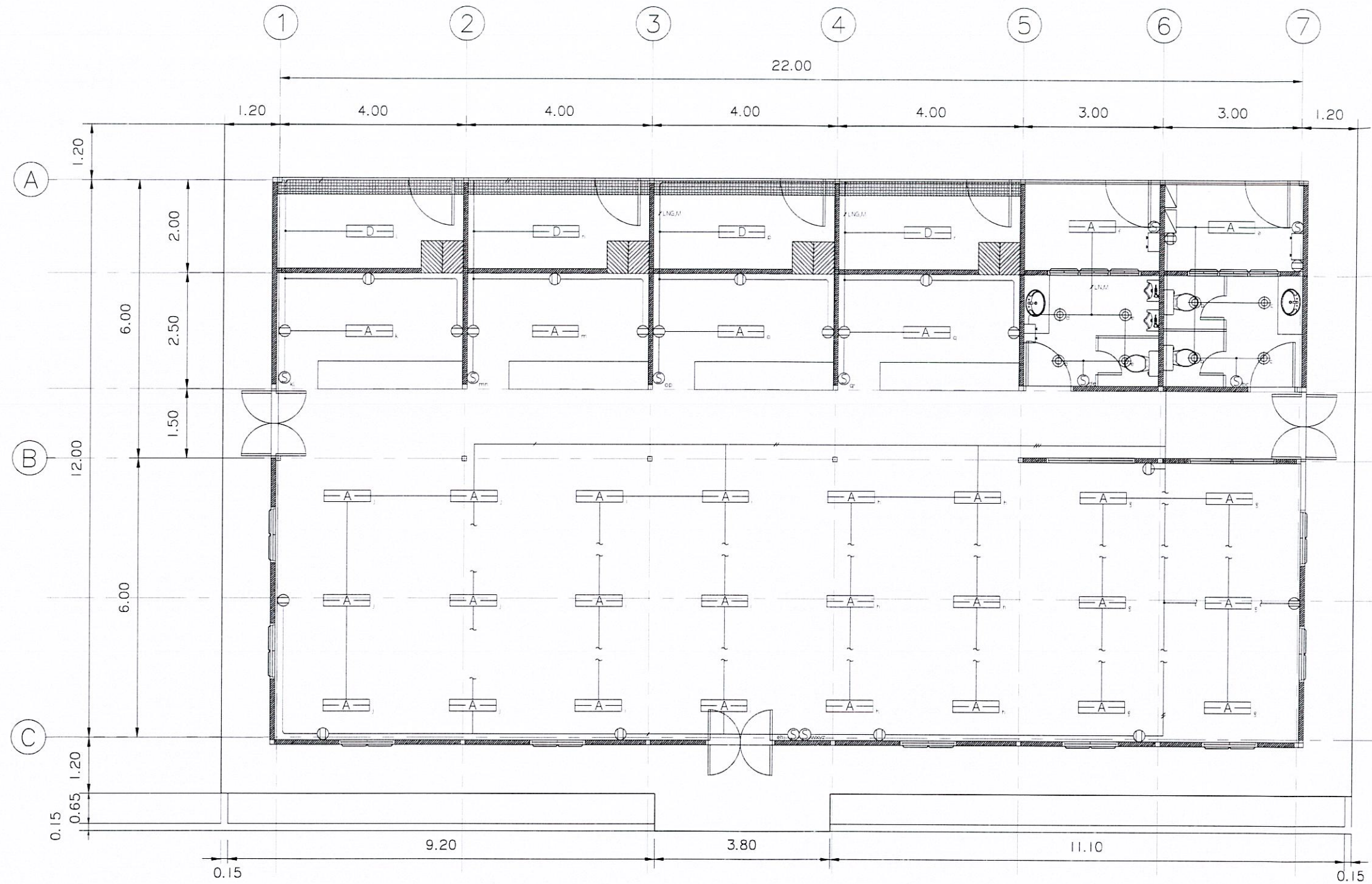
แปลนงานโคมไฟฟ้าแสงสว่างภายใน อาคารโรงอาหารชั่วคราว
