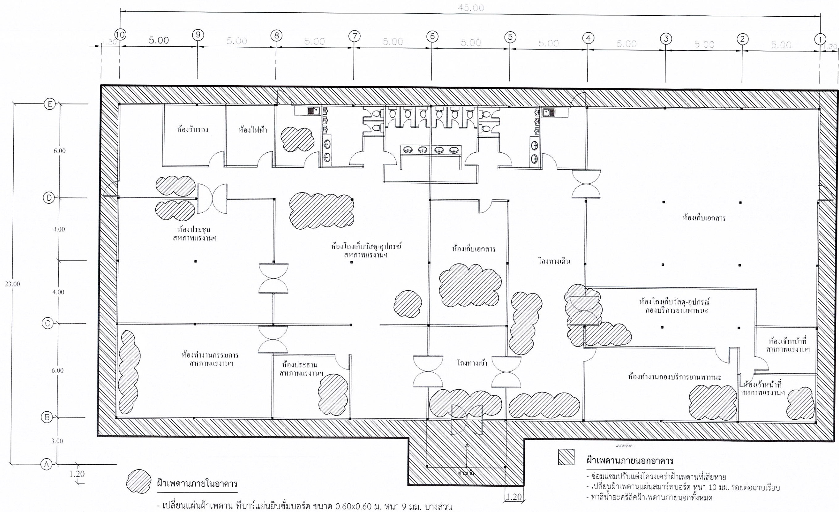
แปลน ฝ้าเพดานภายนอก-ภายใน อาคารที่ทำการสหภาพแรงงานรัฐวิสาหกิจฯ
