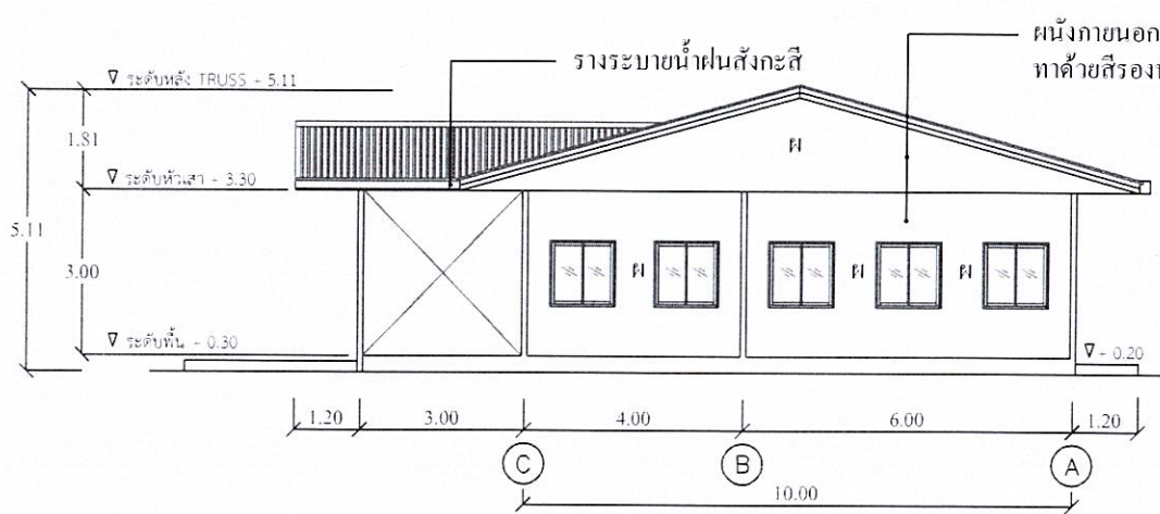
รูปด้าน D อาคารสำนักงานโครงการ 1 : 150
