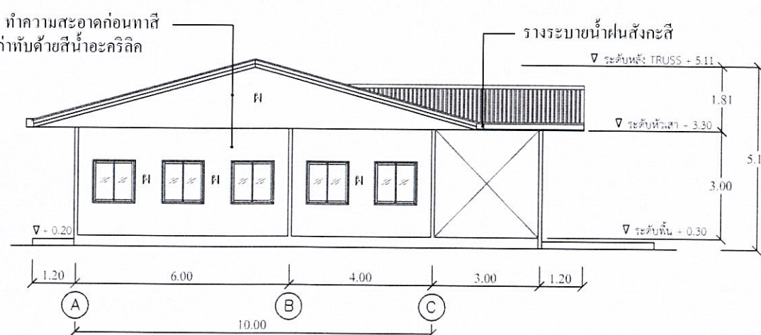
รูปด้าน B อาคารสำนักงานโครงการ 1 : 150
